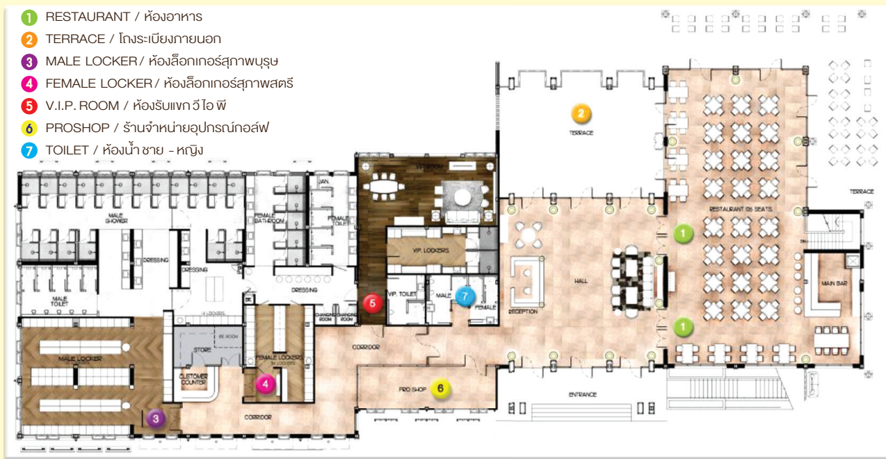
แผนผังคลับเฮาส์ “กรังด์ปรีซ์ กอล์ฟ คลับ”
